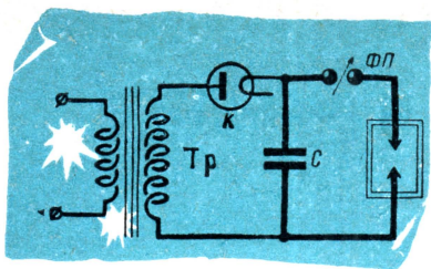
Схема электрогидравлической установки.
