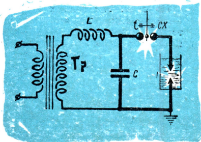
Схема резонансной установки ЭЛГИДЭ.
