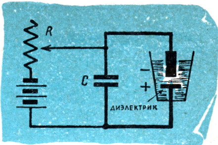
Схема установки электроискровой обработки металлов.
